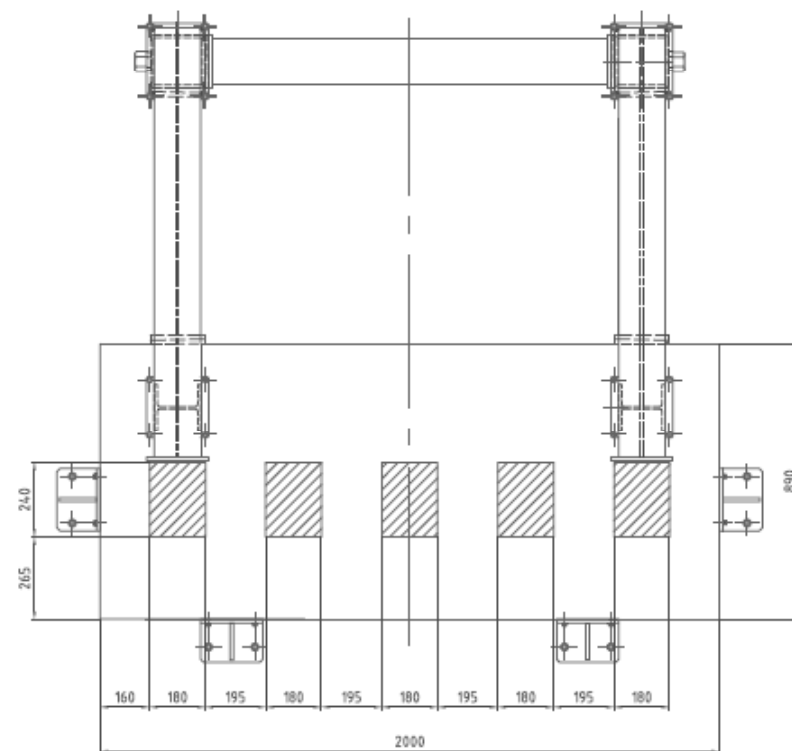
垂直ベンチ下面支持位置
