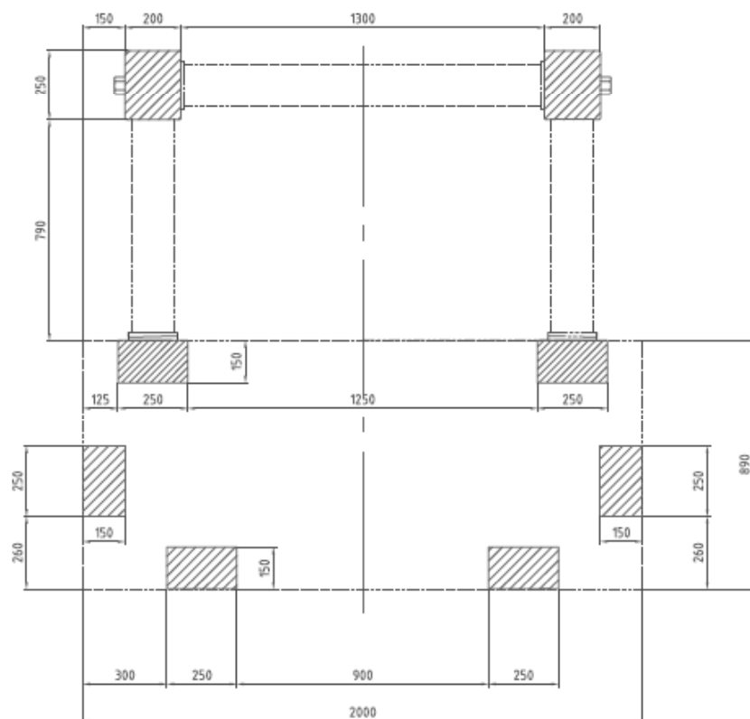
水平架台下面支持位置
